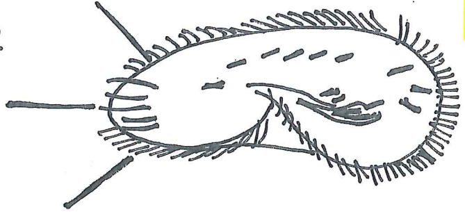
Sphyrapoda
