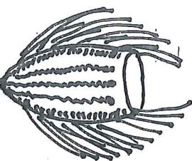
Paramecium (Pantoffeltierchen)
